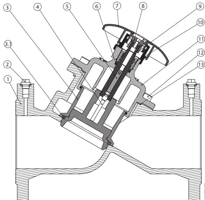
MSV-F2 DN 100-150
