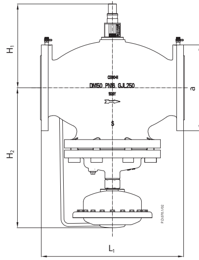
AB-QM DN 150
